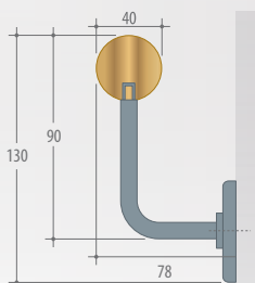
Ménsula de fijación en acero inoxidable
