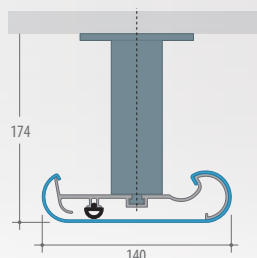
Ménsula de fijación de acero inoxidable
