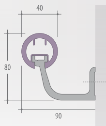
Ménsula de fijación en aluminio
