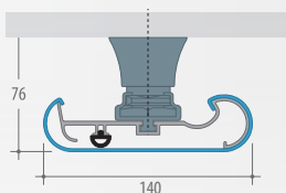
Ménsula de fijación Acrovyn®
