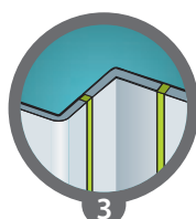
3 Juntas entre ángulos internos y externos
